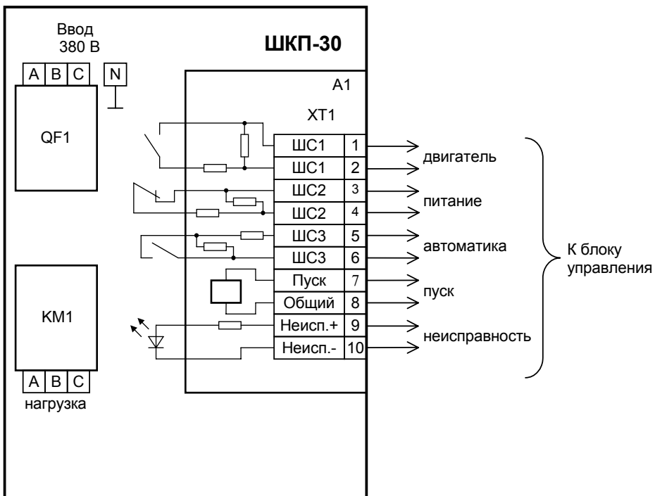
Рисунок 1 Схема электрическая подключения шкафа «ШКП-30» при эксплуатации
