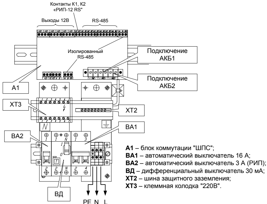
Рисунок 1 Схема расположения основных элементов "ШПС"
