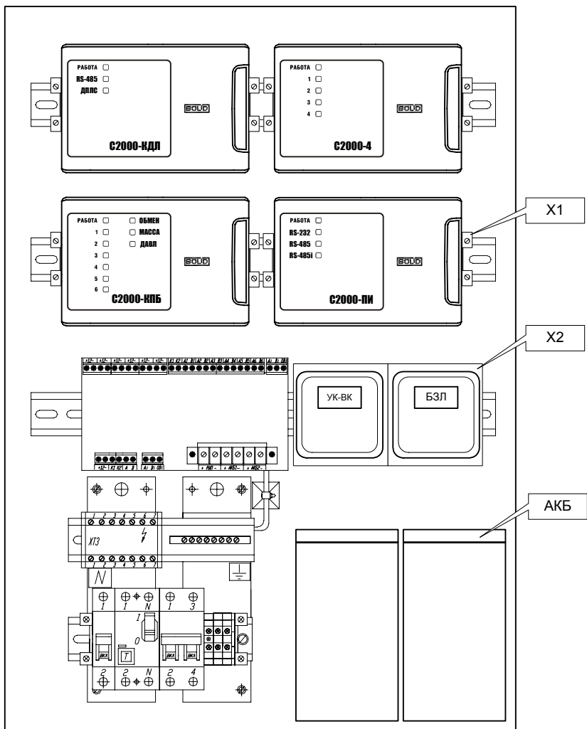
Рисунок 2 Пример компоновки "ШПС"
