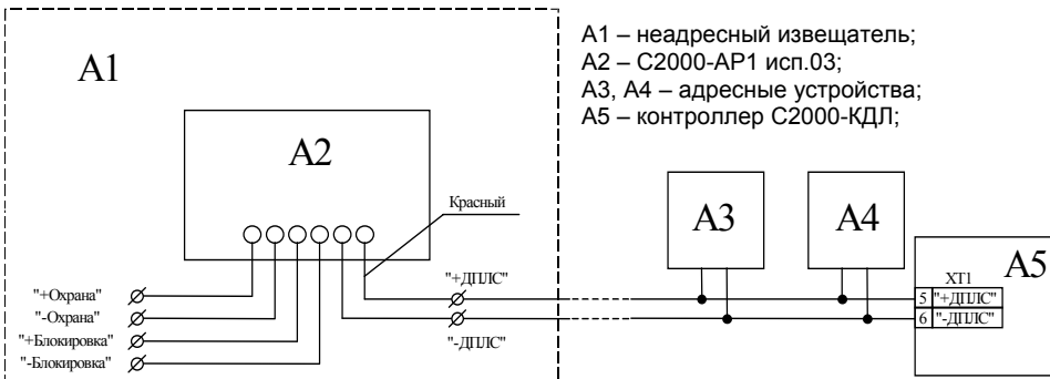
Рис.1 Схема соединений
