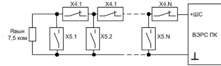
Рис.6. Схема включения охранных извещателей.
