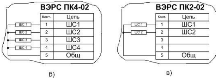
Рис.2. Схемы внешних соединений приборов ВЭРС-ПК(8,4,2)(П,М)(Т)-02.
