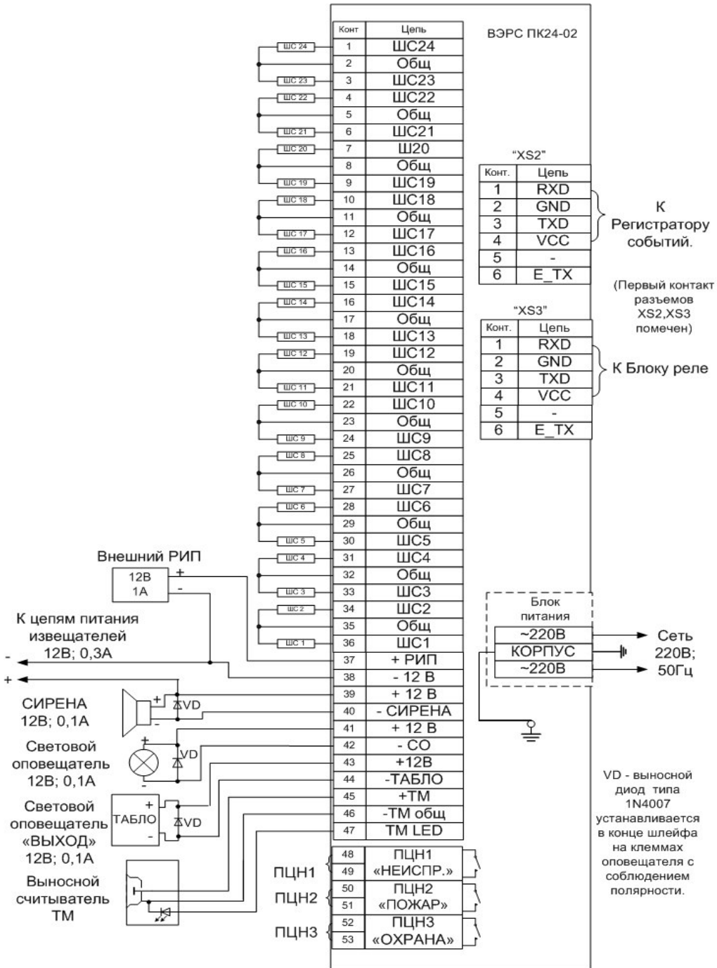
Рис.2. Схема внешних соединений прибора ВЭРС ПК24П-02.
