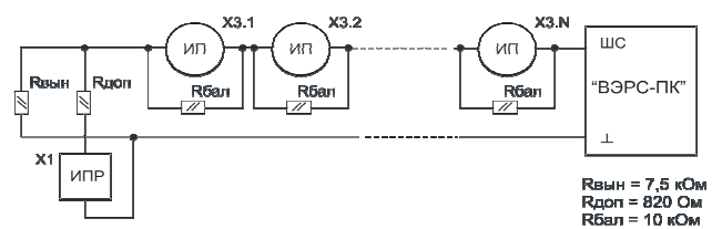
Рис.4. Схемы включения ШС типа ШННС с несколькими тепловыми извещателями (типа ИП-105) и сработкой по двум извещателям (с перезапросом).
