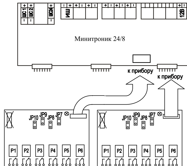
Рис.1. Подключение модуля управления ПР-1 к прибору «Минитроник 24».
