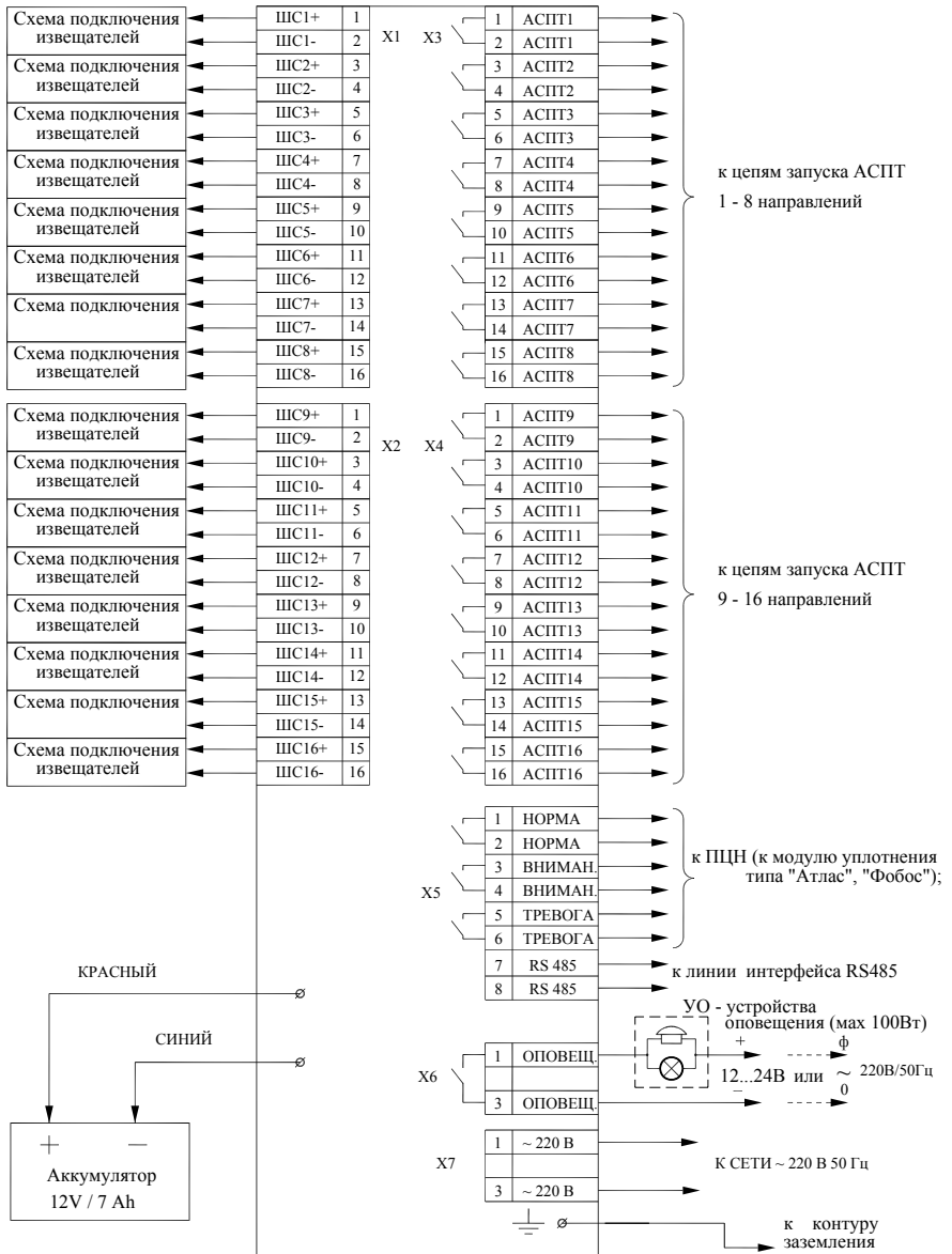
Схема внешних подключений прибора ППКП01149-16-1 "Яхонт-16И"
