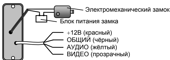
Схема подключения панели JSB
