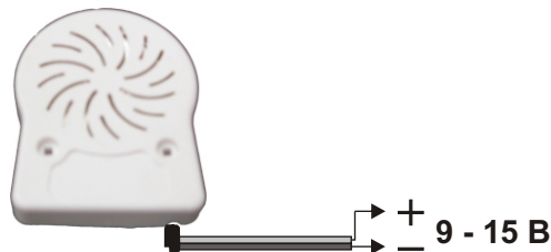
Рис.2 Схема подключения ПКИ-МЦ.
