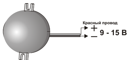
Рис.2 Схема подключения ПКИ - ОС2.
